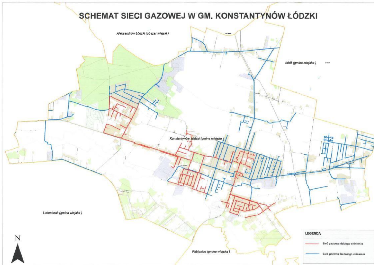
Rysunek 24. Schemat sieci gazowej w Gminie Konstantynów Łódzki [Źródło: dane przekazane przez Polską Spółkę Gazownictwa Sp. z o.o.]
